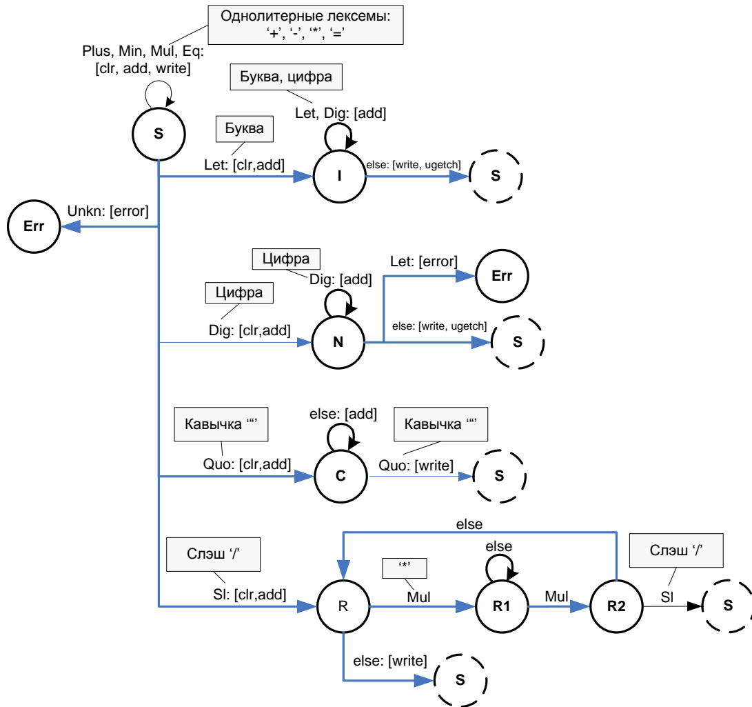
Рис. 5. Фрагмент сканера с процедурной частью
