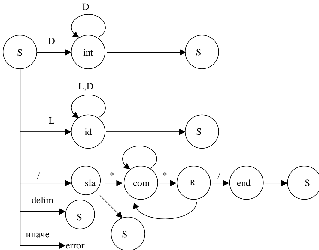
Рис. 4. Упрощенная структура лексического анализатора
