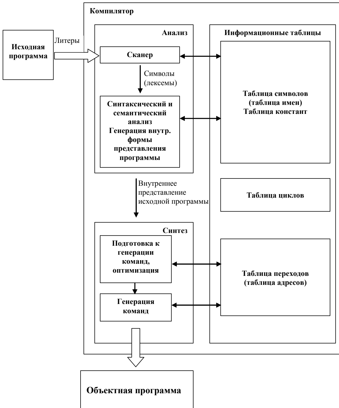
Рис. 1. Структура компилятора
