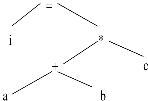
Рис. 2. Дерево выражения i=(a+b)*c
